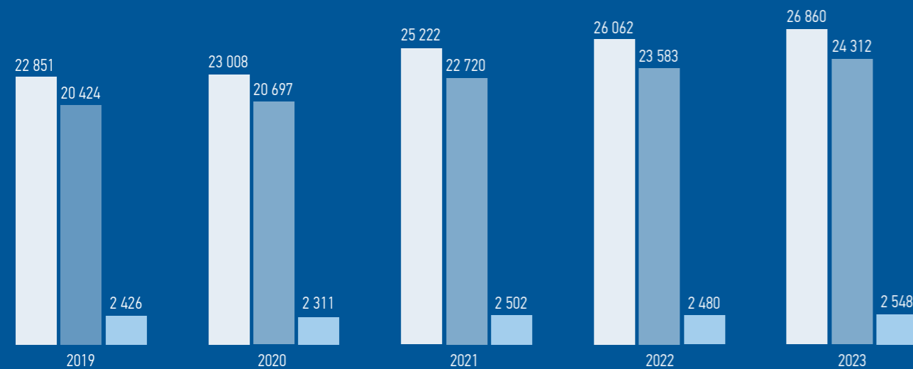
Отпуск электроэнергии в сеть / из сети ПАО «Россети Кубань» и потери при передаче электроэнергии (млн кВт • ч)
